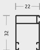
2 Guía Lateral
